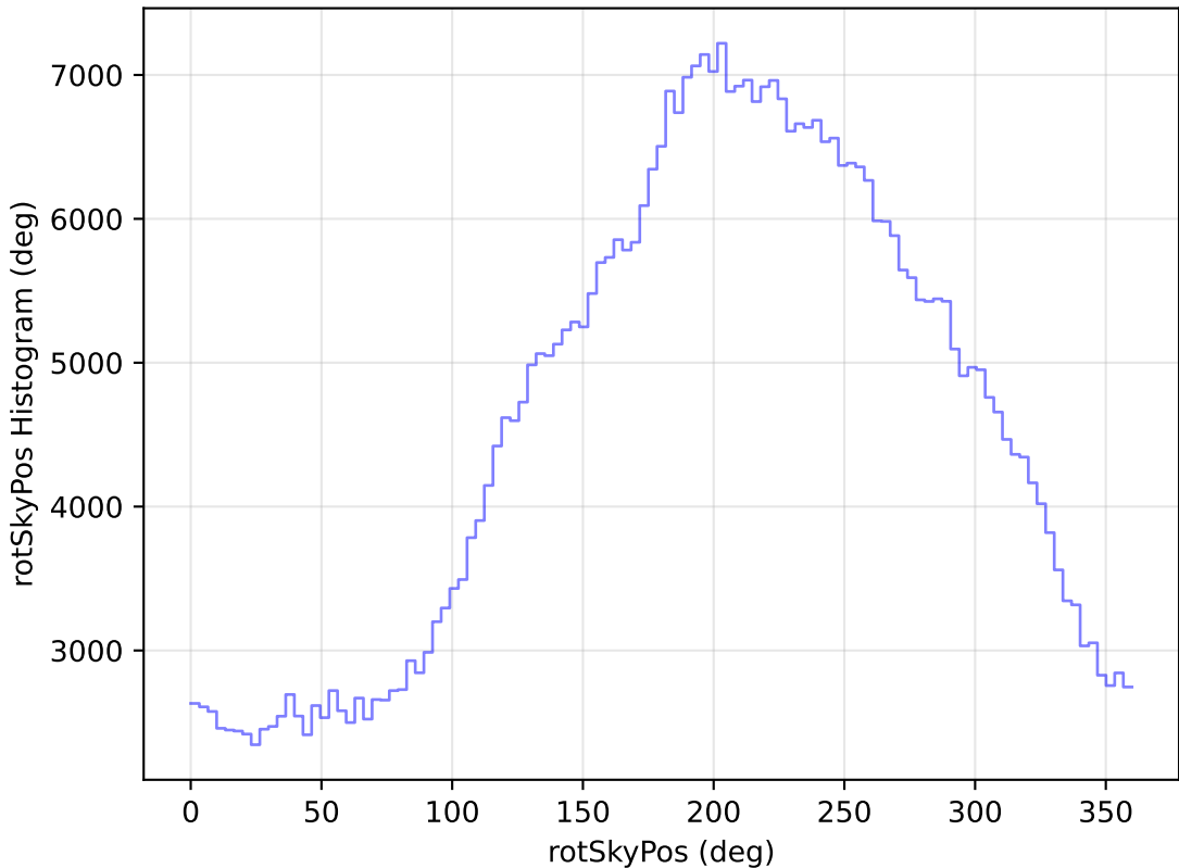
no_magell_roll_v3.4_10yrs All sky i band: rotSkyPos Histogram
