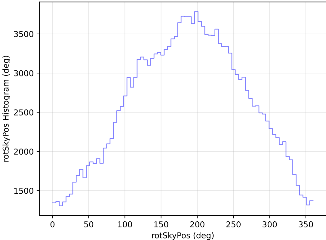
no_magell_roll_v3.4_10yrs All sky g band: rotSkyPos Histogram
