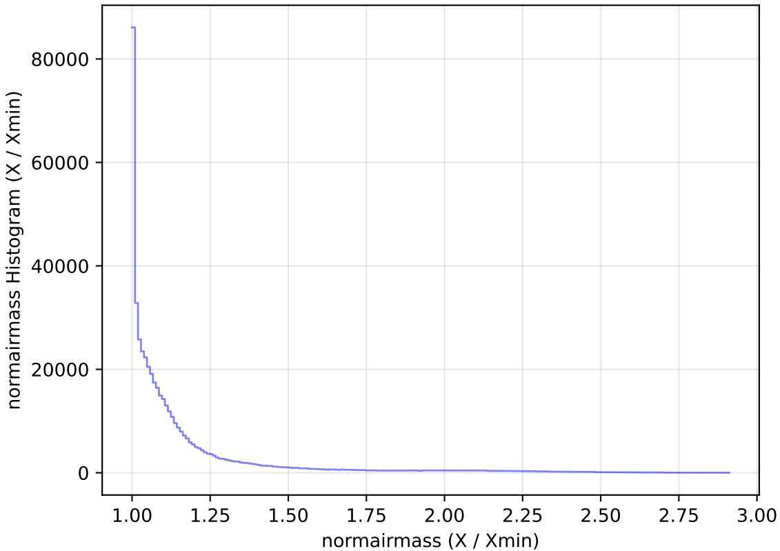
no_magell_roll_v3.4_10yrs WFD i band: normairmass Histogram
