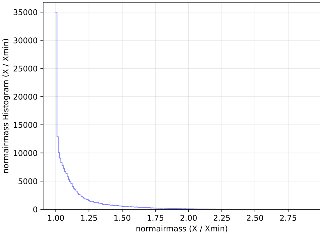
no_magell_roll_v3.4_10yrs WFD g band: normairmass Histogram
