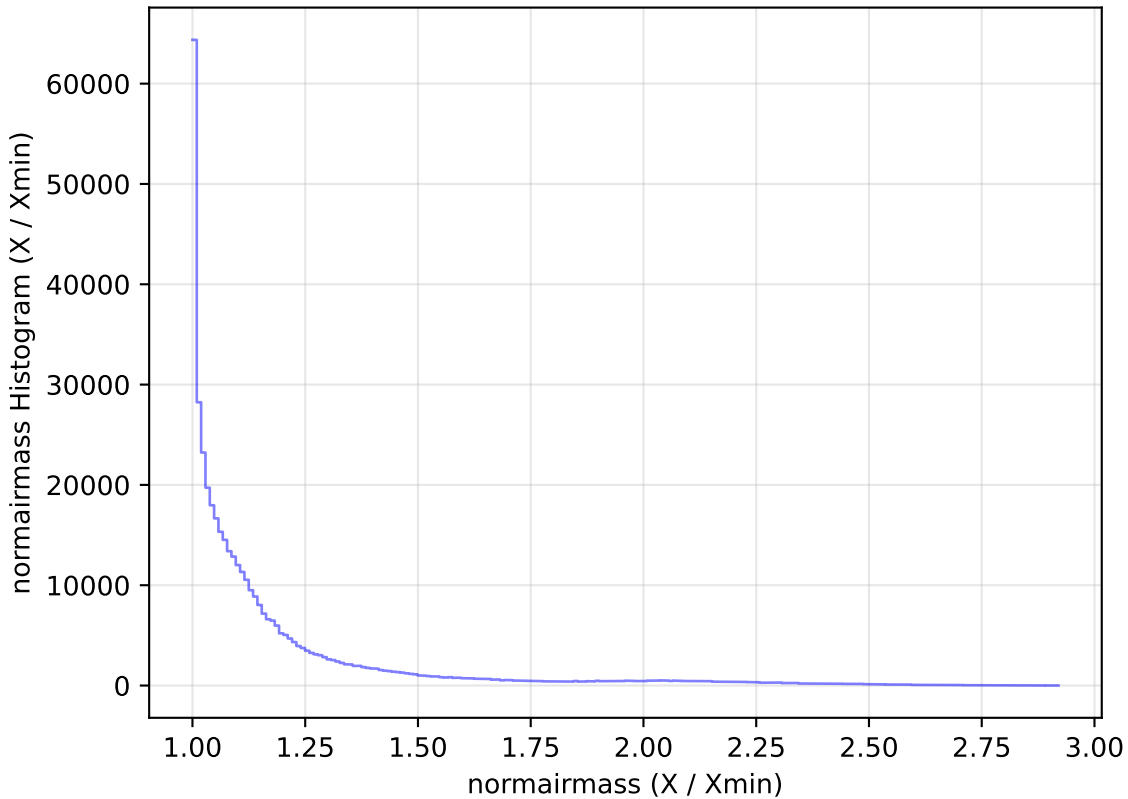
no_magell_roll_v3.4_10yrs All sky z band: normairmass Histogram
