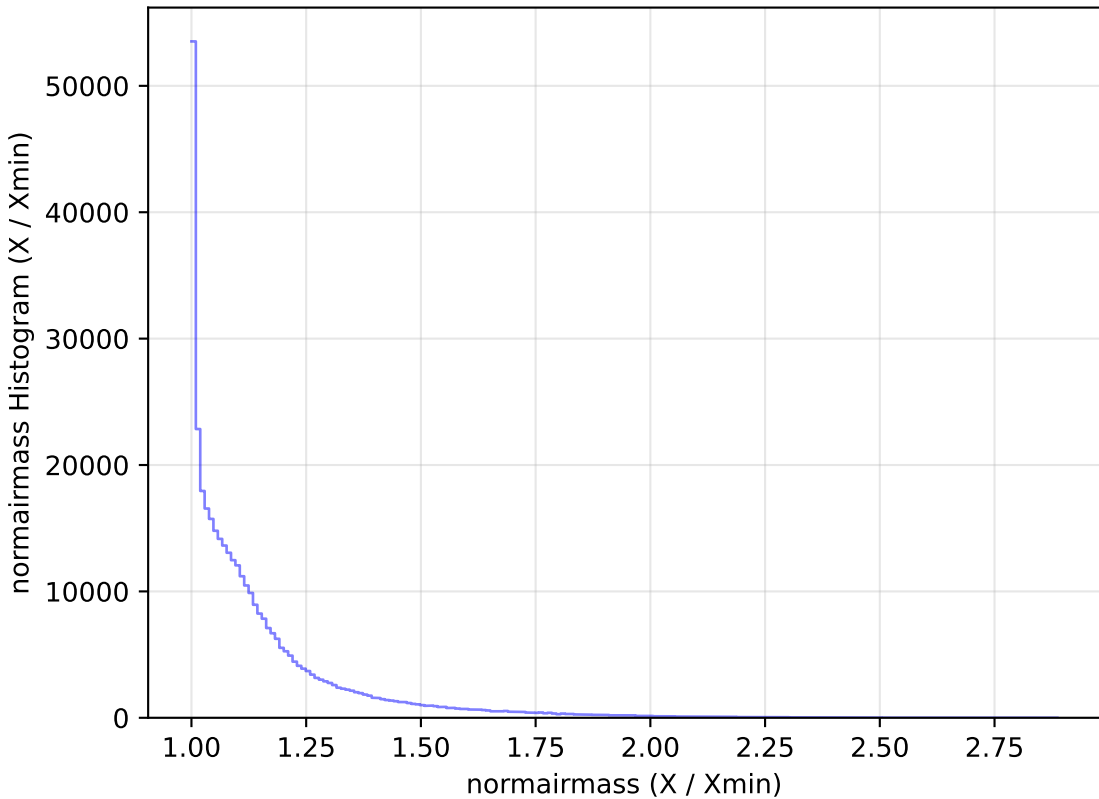
no_magell_roll_v3.4_10yrs All sky y band: normairmass Histogram
