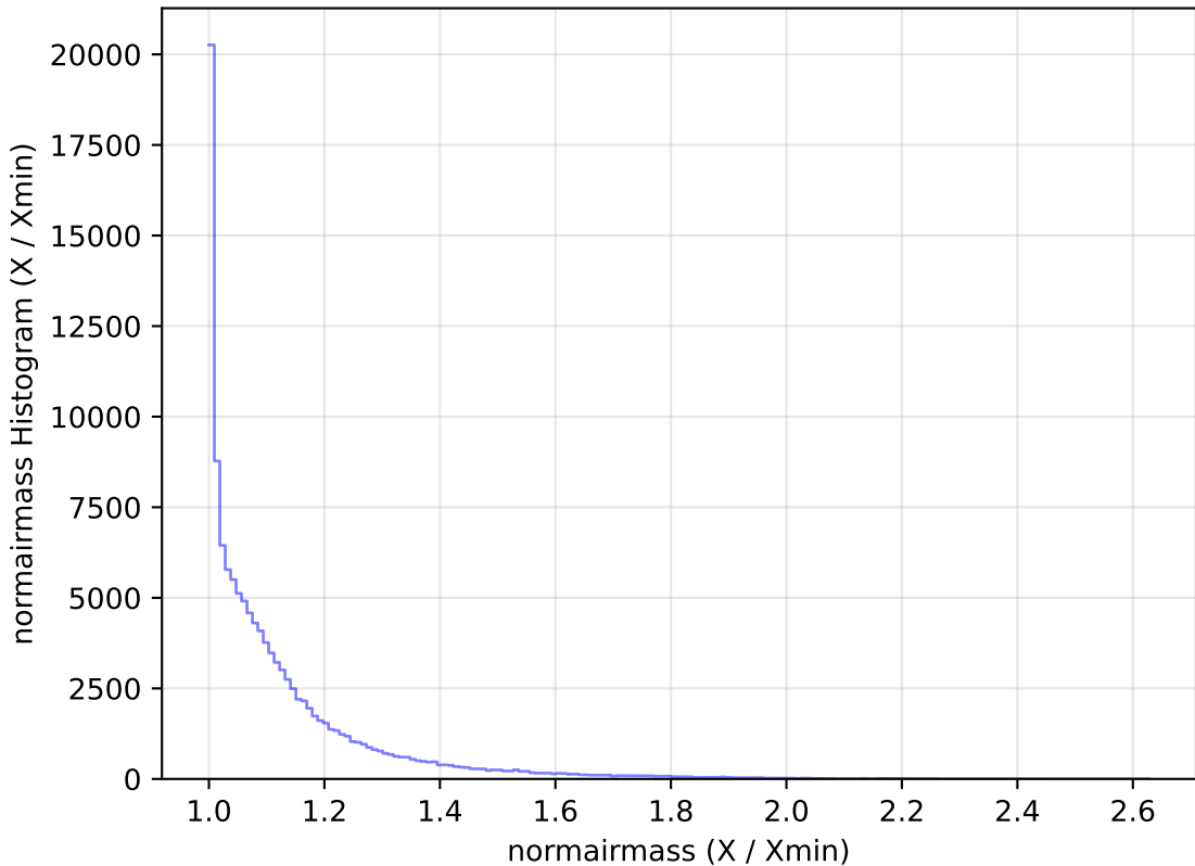
no_magell_roll_v3.4_10yrs All sky u band: normairmass Histogram
