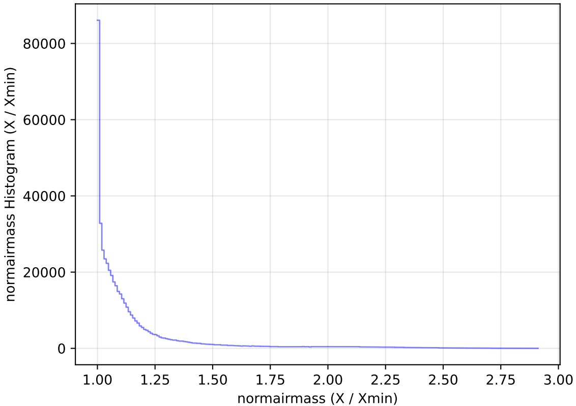
no_magell_roll_v3.4_10yrs All sky i band: normairmass Histogram
