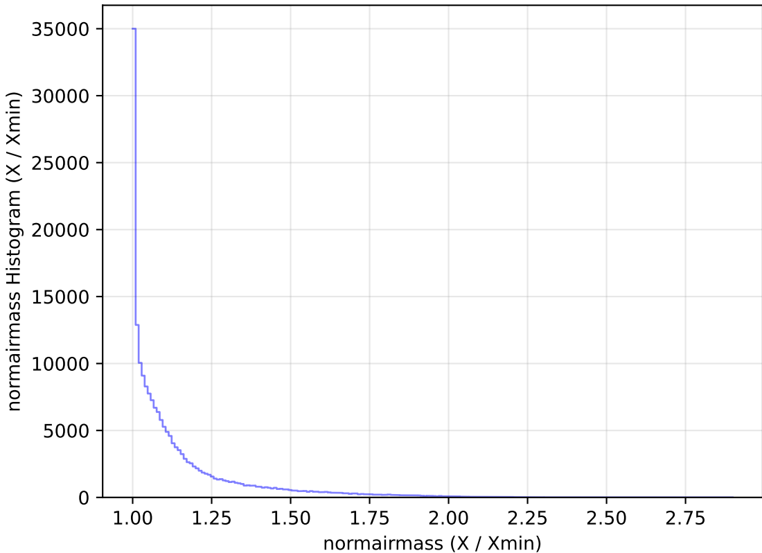
no_magell_roll_v3.4_10yrs All sky g band: normairmass Histogram
