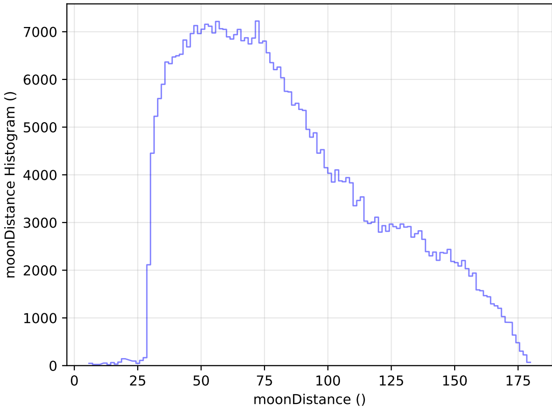
no_magell_roll_v3.4_10yrs WFD z band: moonDistance Histogram
