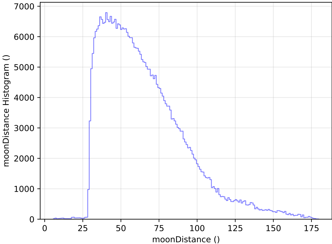
no_magell_roll_v3.4_10yrs WFD y band: moonDistance Histogram
