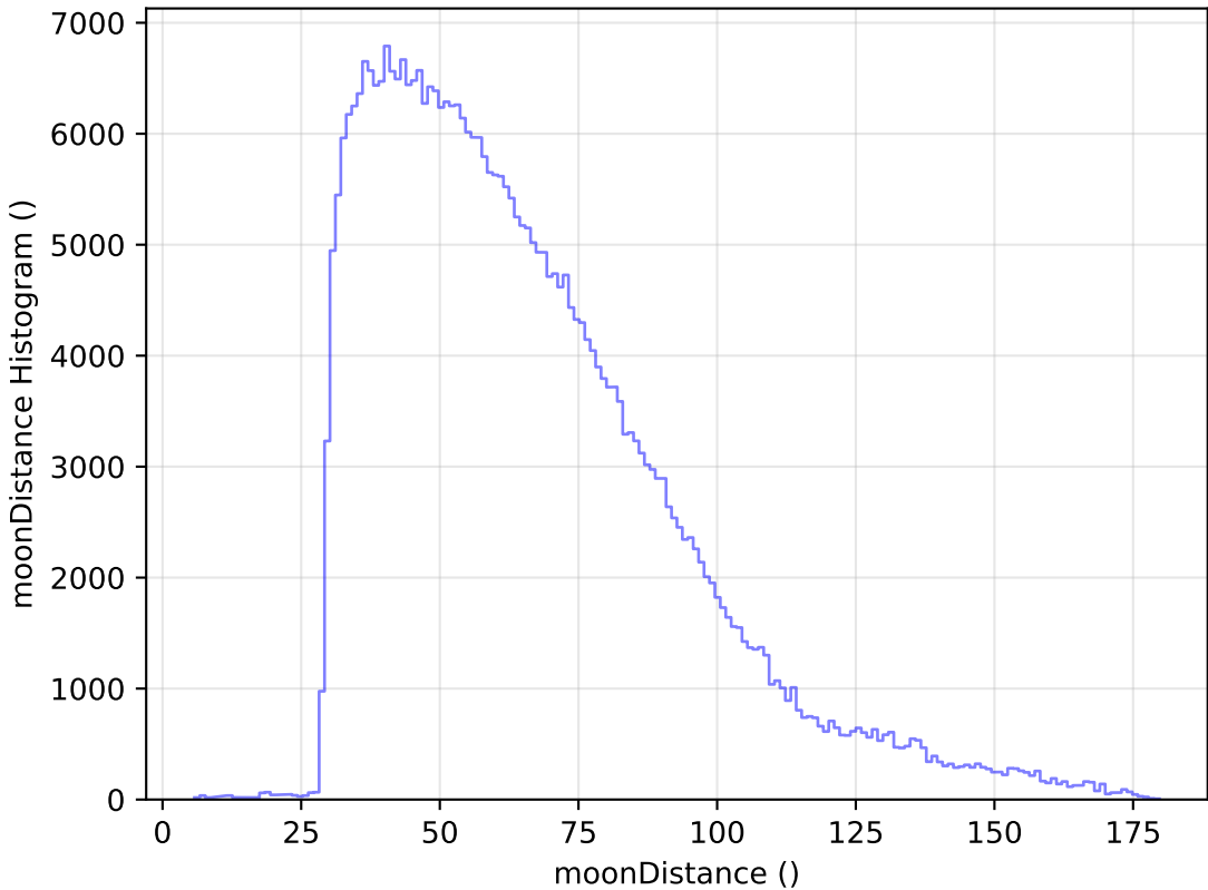
no_magell_roll_v3.4_10yrs All sky y band: moonDistance Histogram
