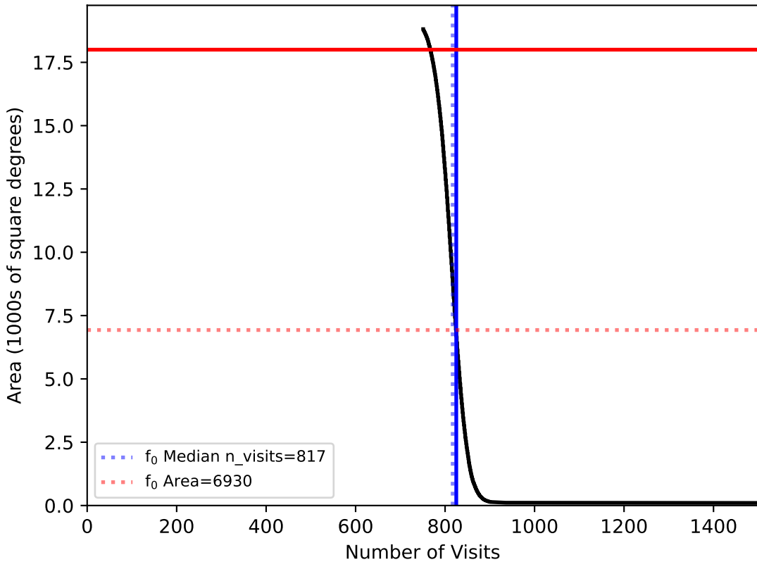
no_magell_roll_v3.4_10yrs WFD: f0
