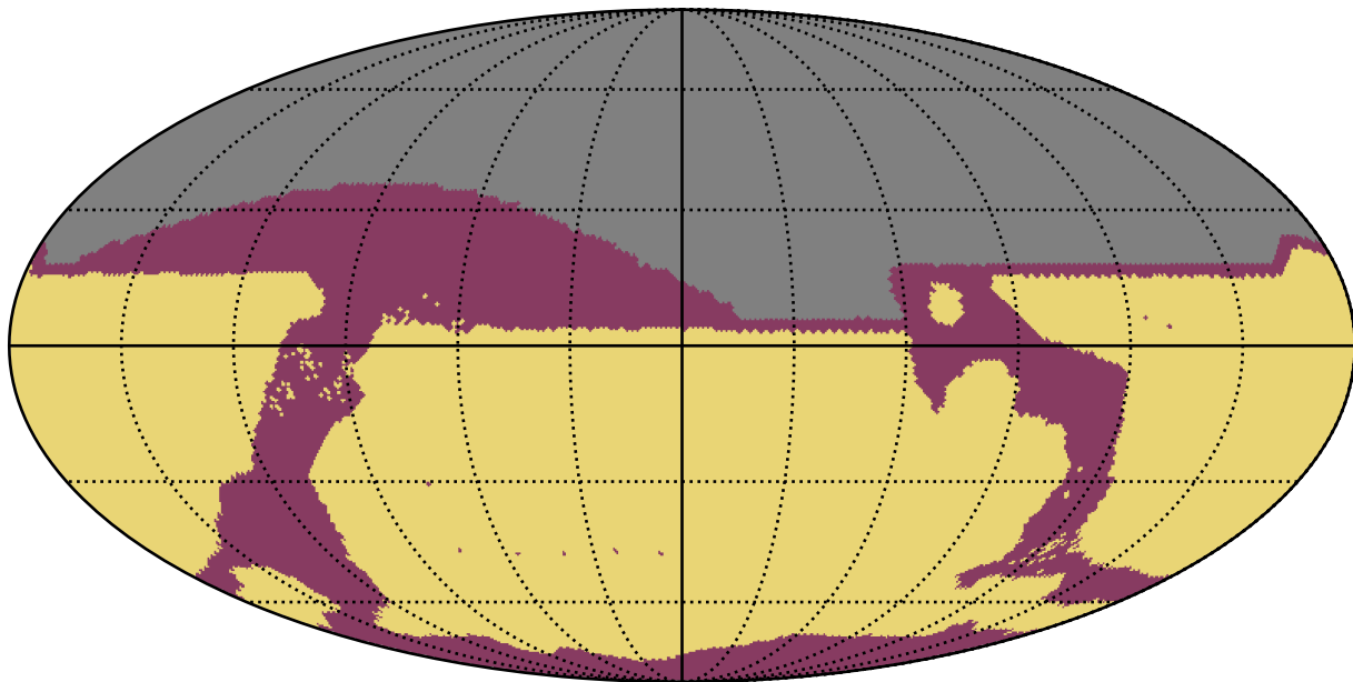
no_magell_roll_v3.4_10yrs All sky: RapidRevisits
