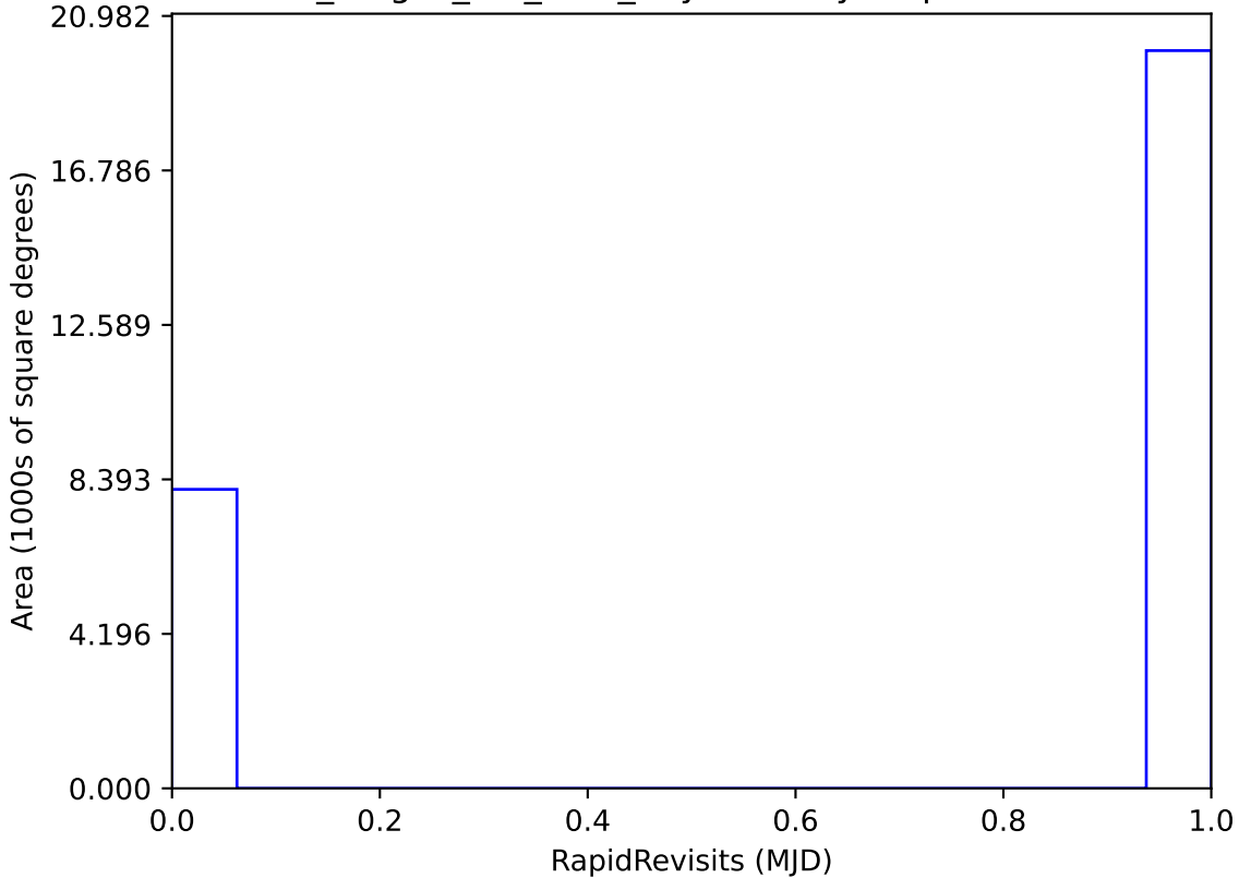
no_magell_roll_v3.4_10yrs All sky: RapidRevisits
