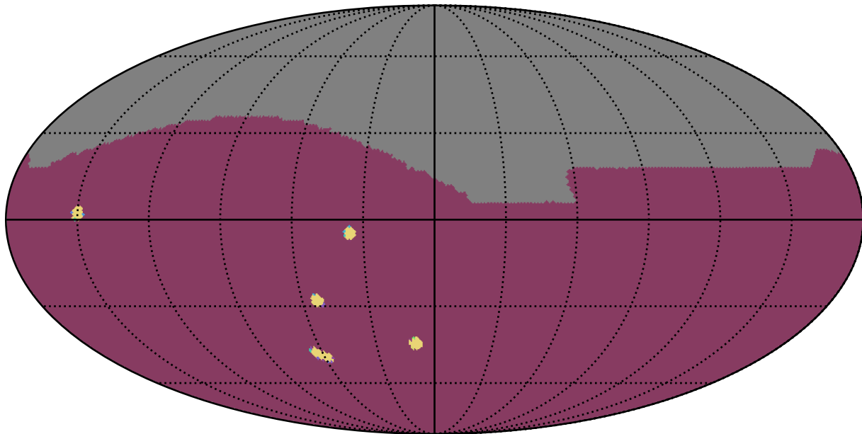
no_magell_roll_v3.4_10yrs All sky: NumberOfQuickRevisits
