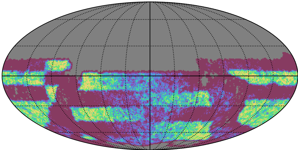
no_magell_roll_v3.4_10yrs Yr 3-4 y band: NVisits
