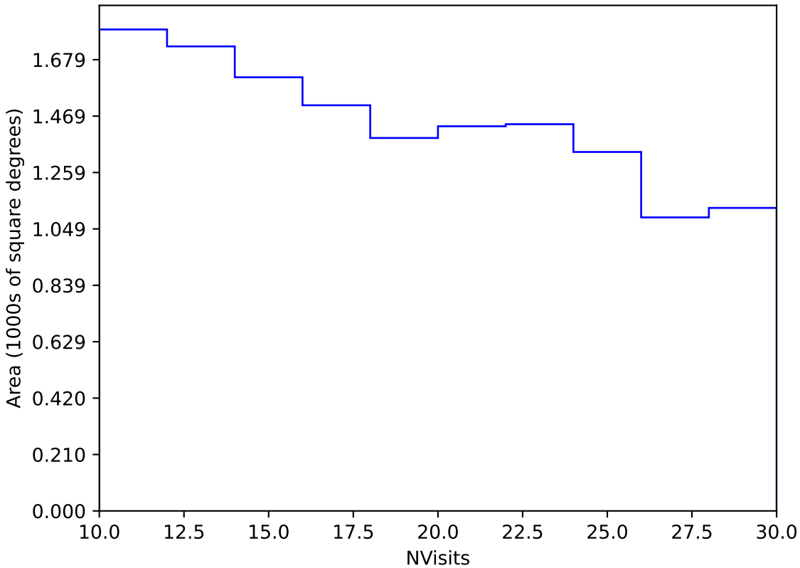
no_magell_roll_v3.4_10yrs Yr 3-4 y band: NVisits
