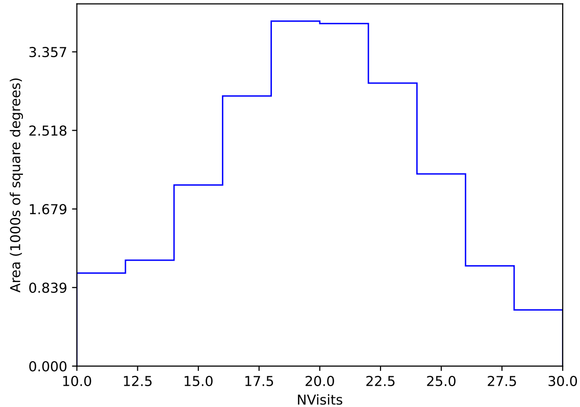
no_magell_roll_v3.4_10yrs Yr 1 y band: NVisits
