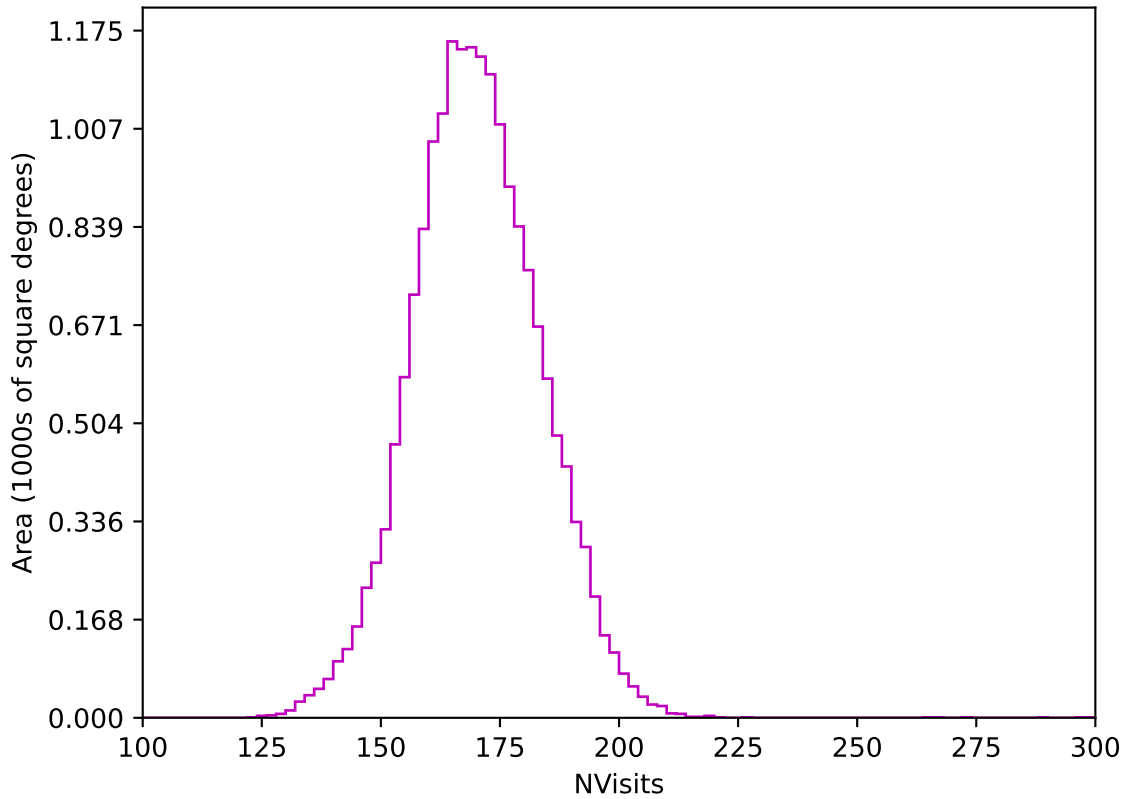
no_magell_roll_v3.4_10yrs WFD z band: NVisits
