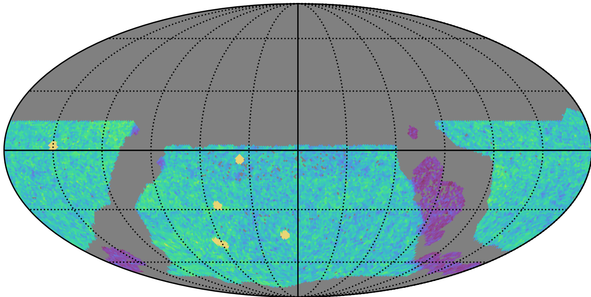
no_magell_roll_v3.4_10yrs WFD u band: NVisits
