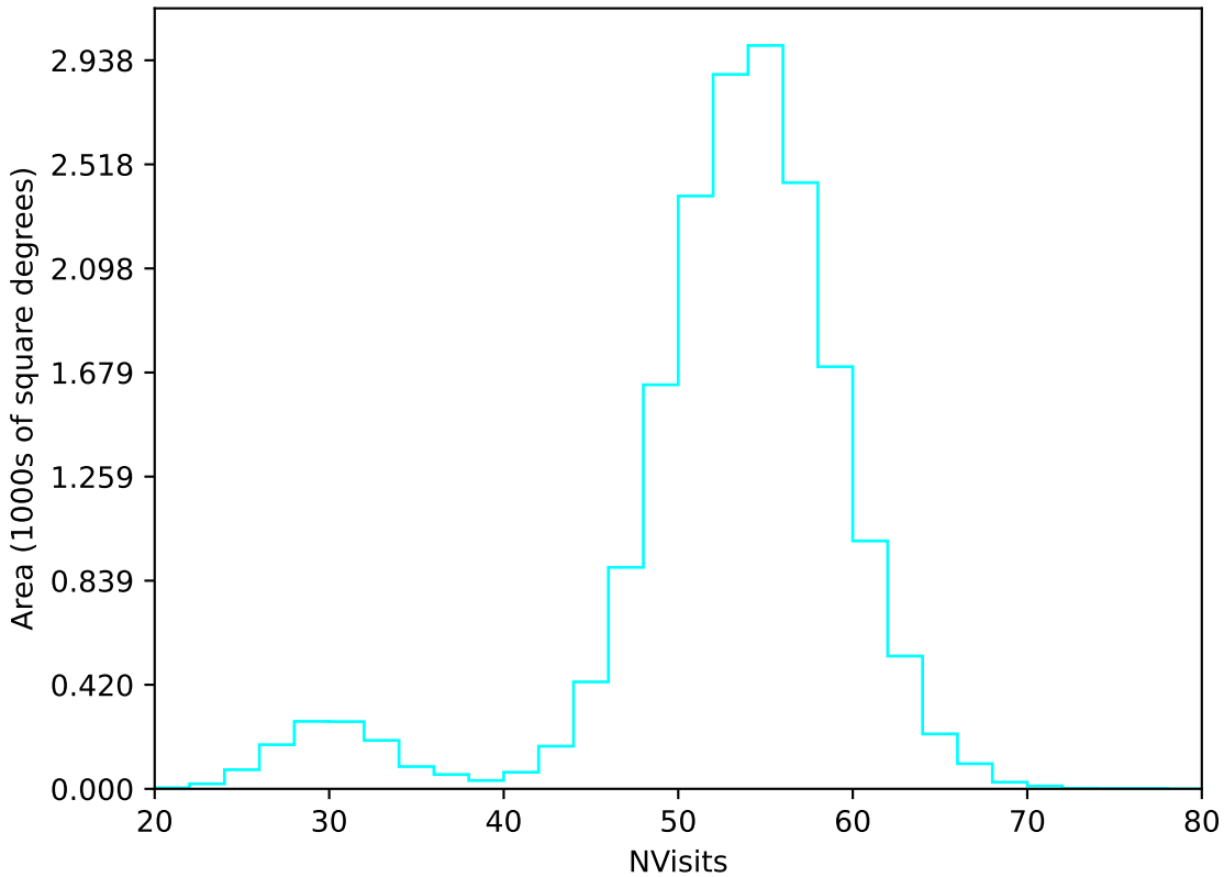
no_magell_roll_v3.4_10yrs WFD u band: NVisits
