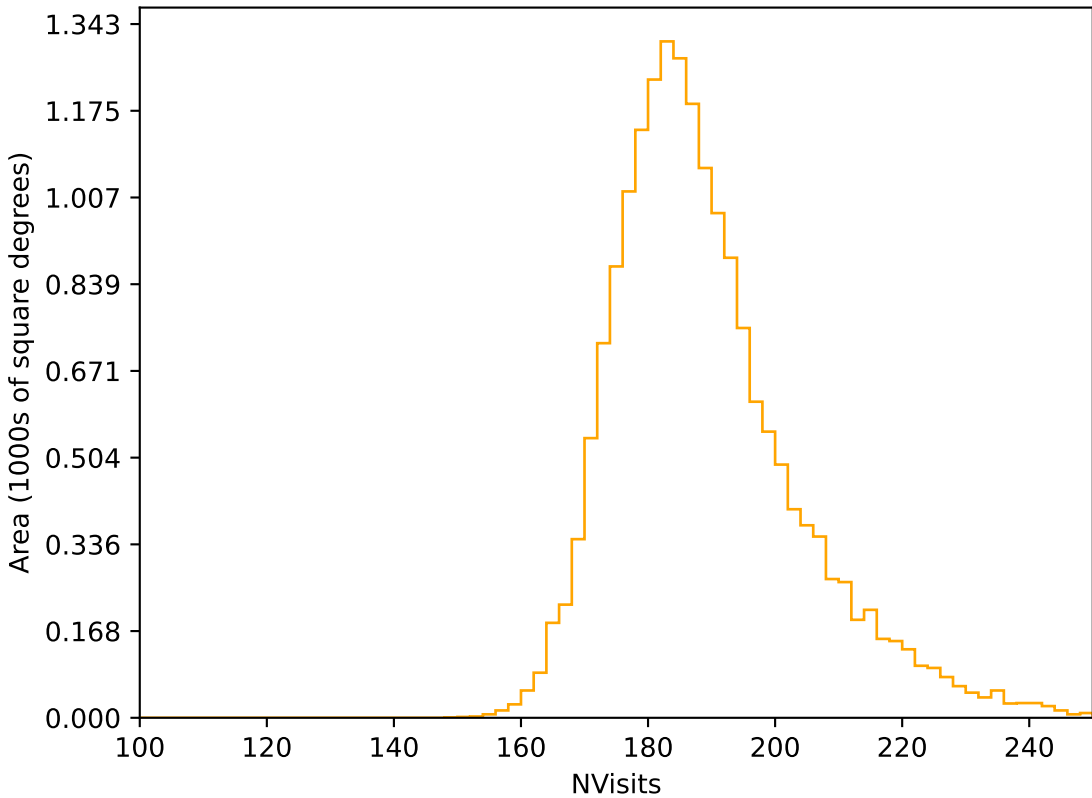
no_magell_roll_v3.4_10yrs WFD r band: NVisits
