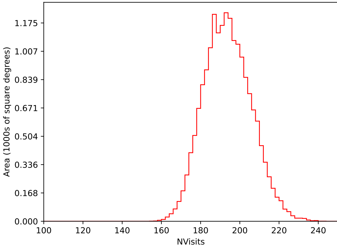
no_magell_roll_v3.4_10yrs WFD i band: NVisits
