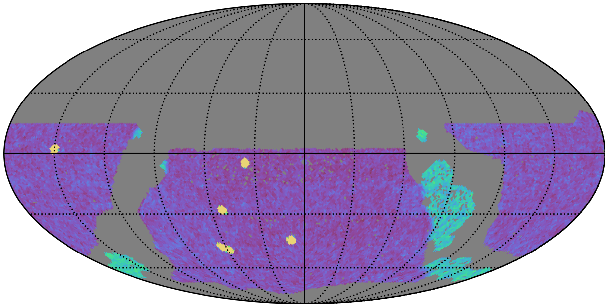
no_magell_roll_v3.4_10yrs WFD g band: NVisits
