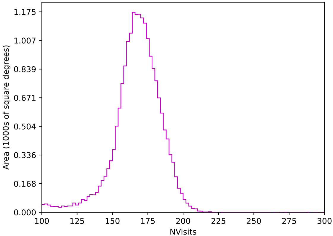
no_magell_roll_v3.4_10yrs All sky z band: NVisits
