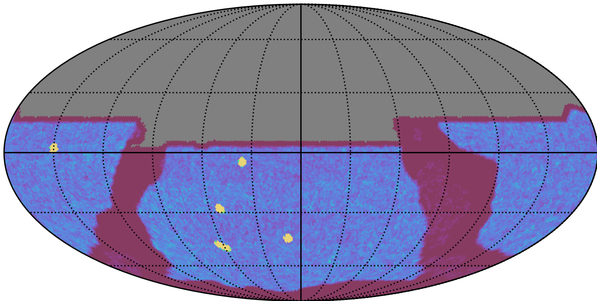
no_magell_roll_v3.4_10yrs All sky y band: NVisits
