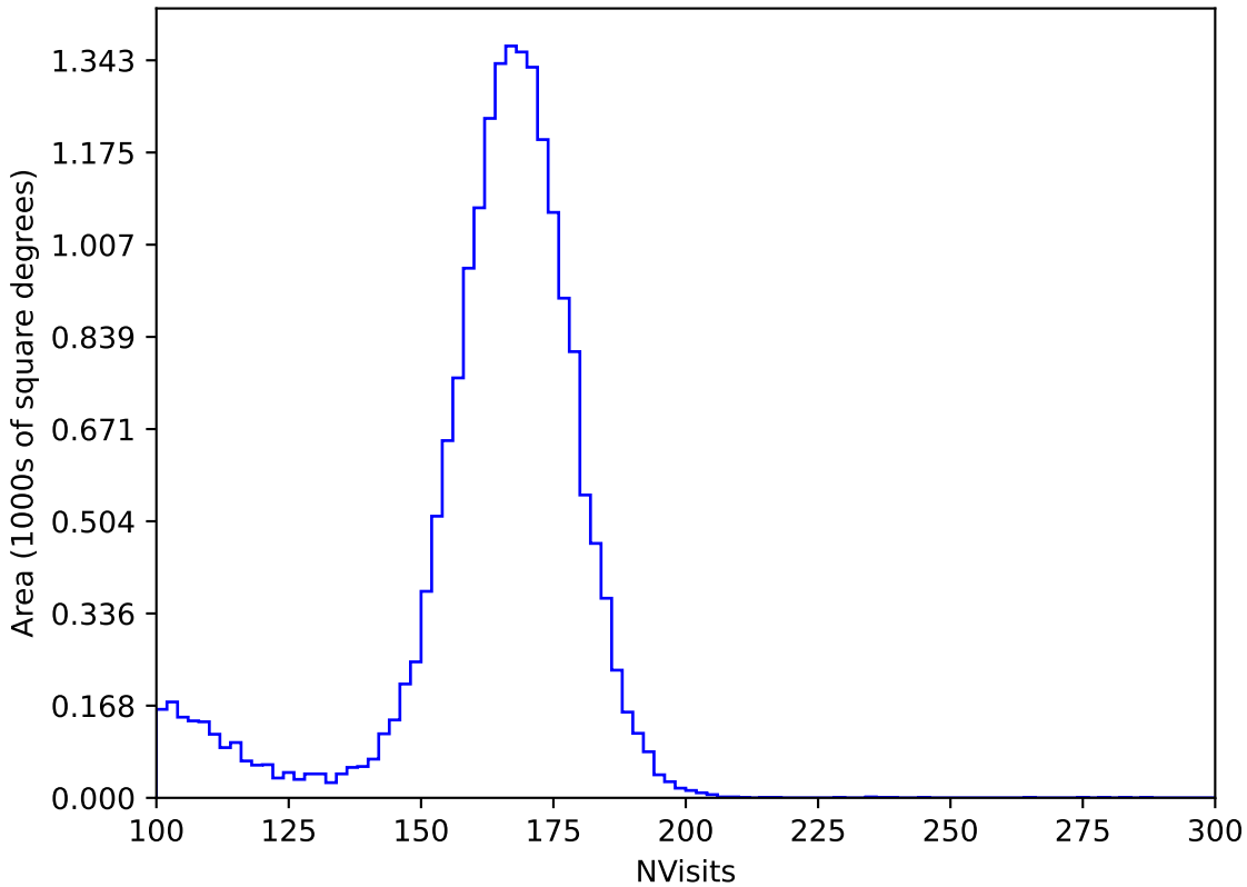
no_magell_roll_v3.4_10yrs All sky y band: NVisits
