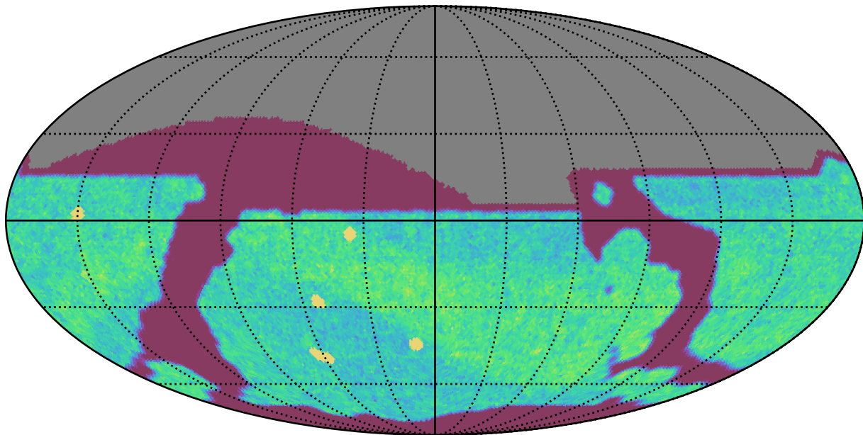
no_magell_roll_v3.4_10yrs All sky i band: NVisits
