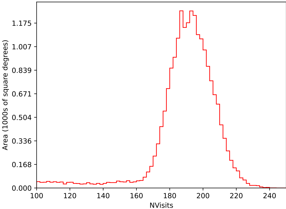
no_magell_roll_v3.4_10yrs All sky i band: NVisits
