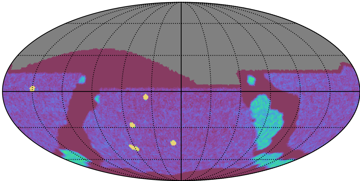
no_magell_roll_v3.4_10yrs All sky g band: NVisits
