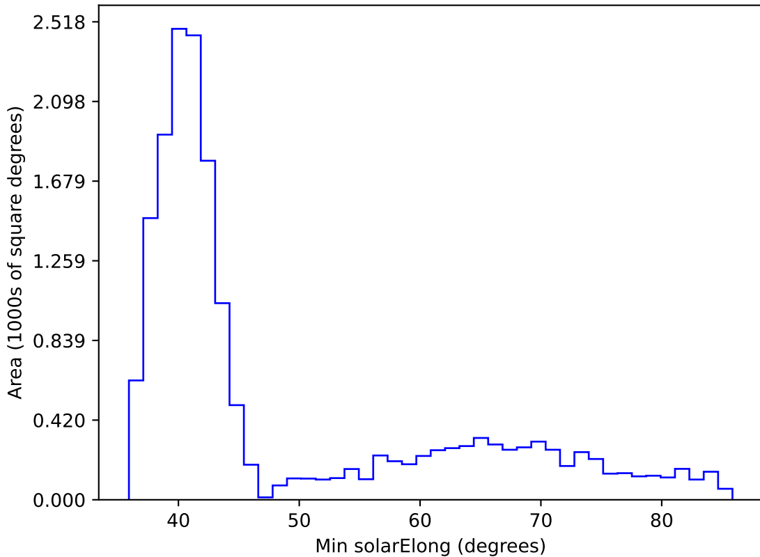
no_magell_roll_v3.4_10yrs WFD z band: Min solarElong
