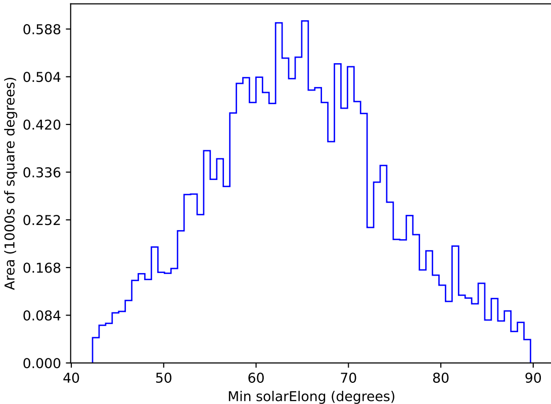
no_magell_roll_v3.4_10yrs WFD y band: Min solarElong
