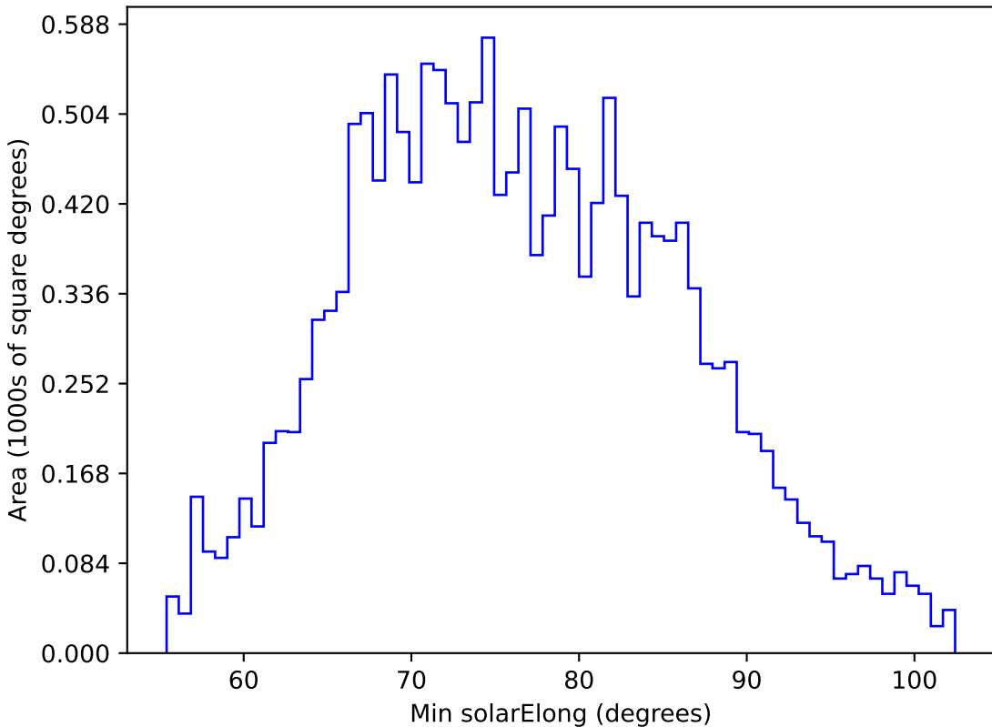
no_magell_roll_v3.4_10yrs WFD u band: Min solarElong
