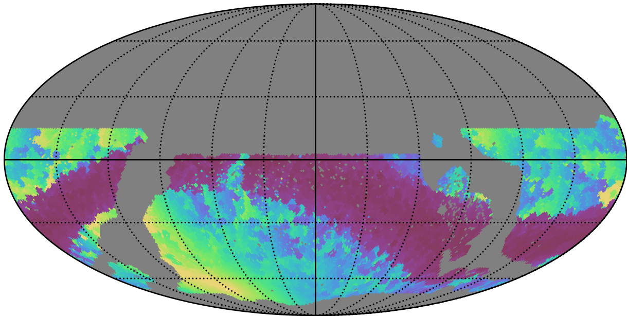
no_magell_roll_v3.4_10yrs WFD r band: Min solarElong
