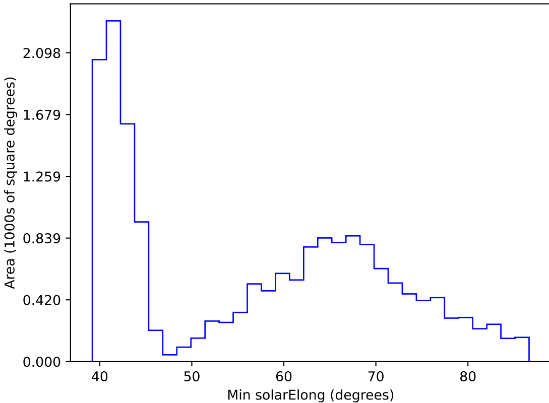
no_magell_roll_v3.4_10yrs WFD r band: Min solarElong
