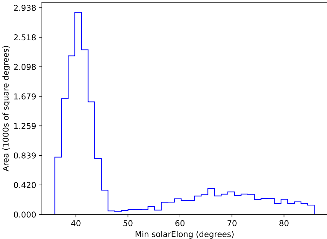
no_magell_roll_v3.4_10yrs WFD i band: Min solarElong
