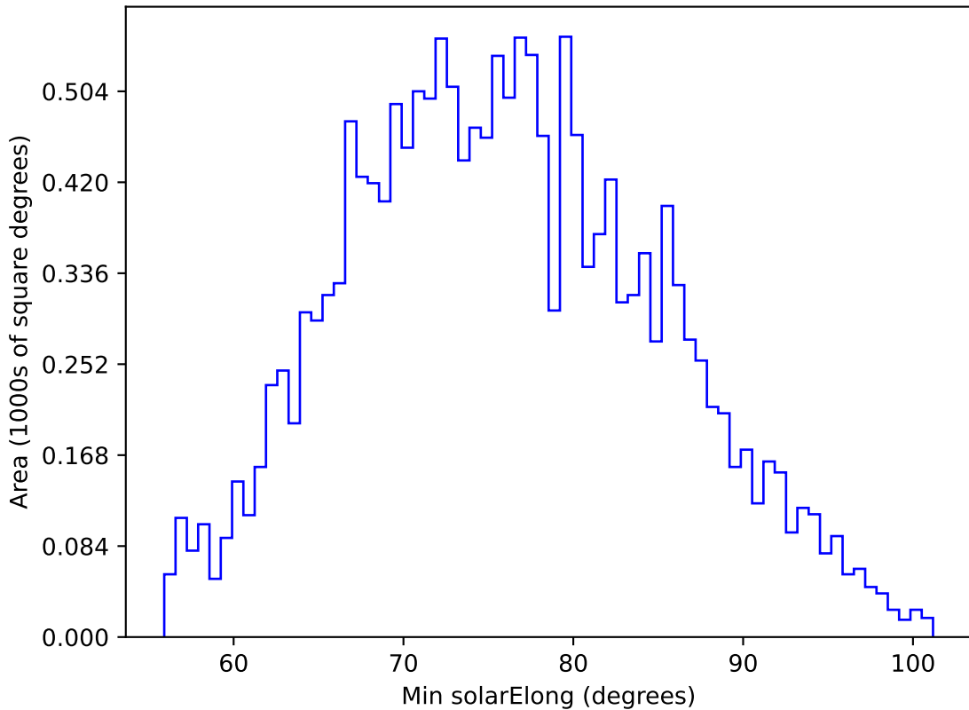
no_magell_roll_v3.4_10yrs WFD g band: Min solarElong
