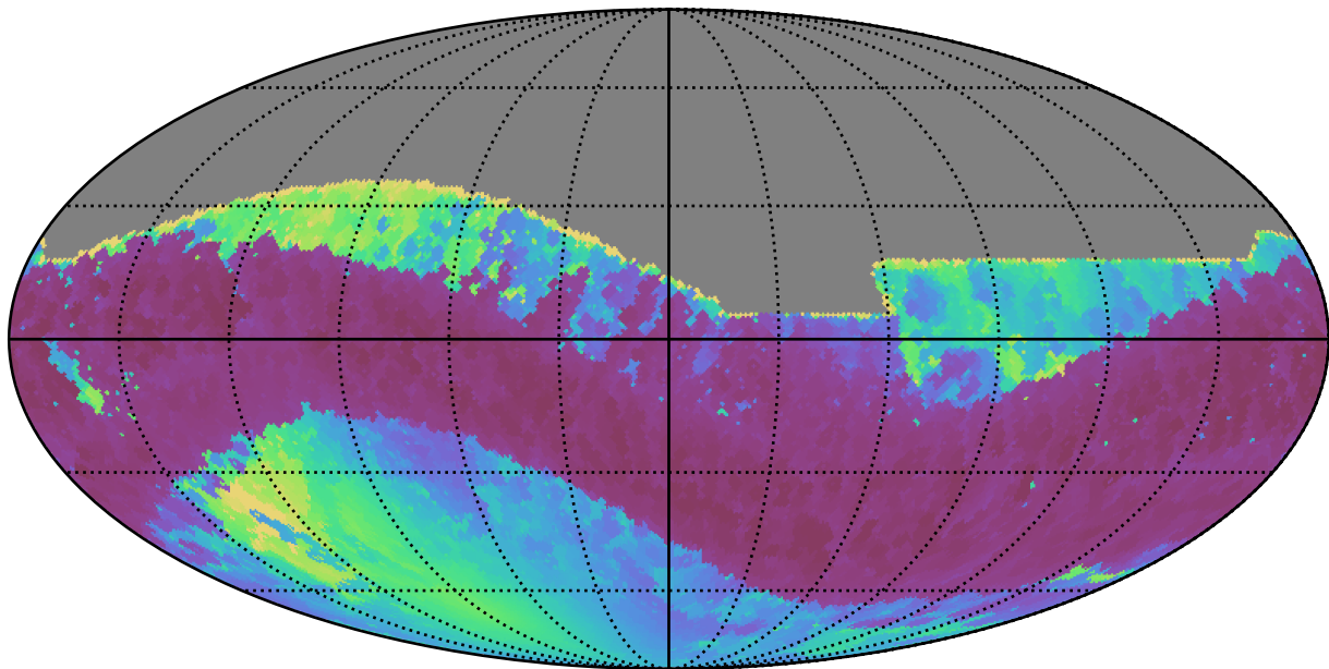
no_magell_roll_v3.4_10yrs All sky z band: Min solarElong
