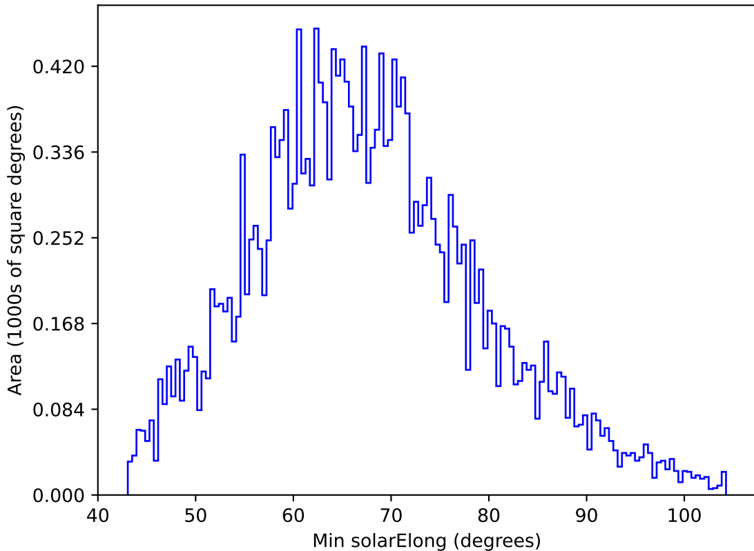
no_magell_roll_v3.4_10yrs All sky y band: Min solarElong
