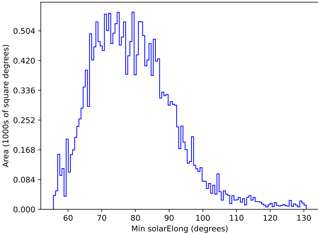
no_magell_roll_v3.4_10yrs All sky u band: Min solarElong
