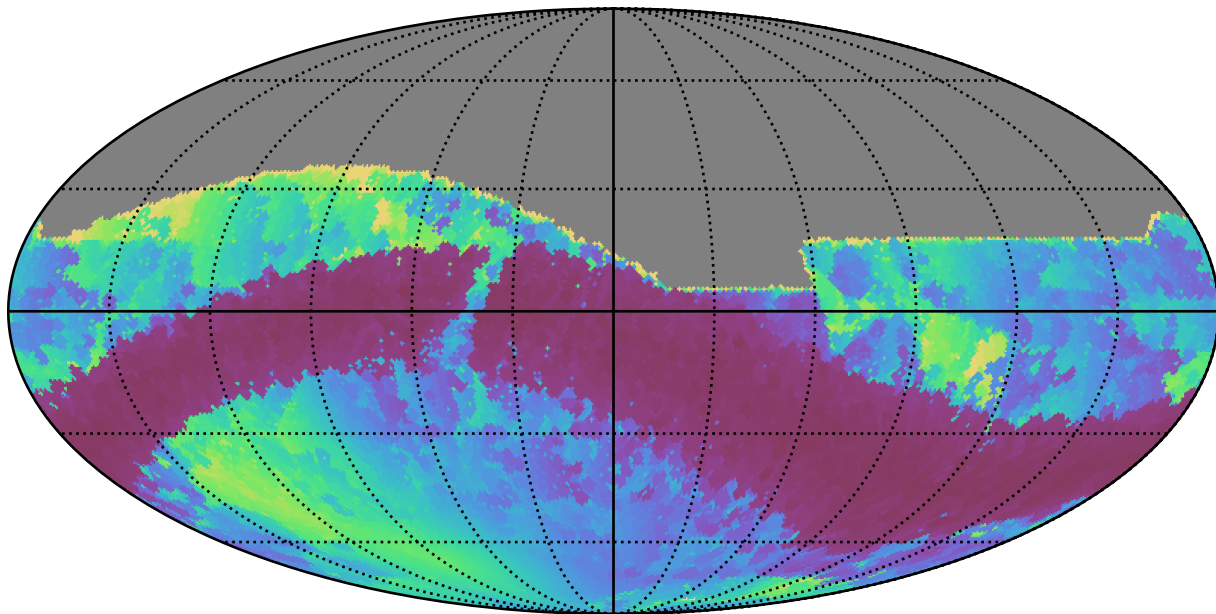
no_magell_roll_v3.4_10yrs All sky r band: Min solarElong
