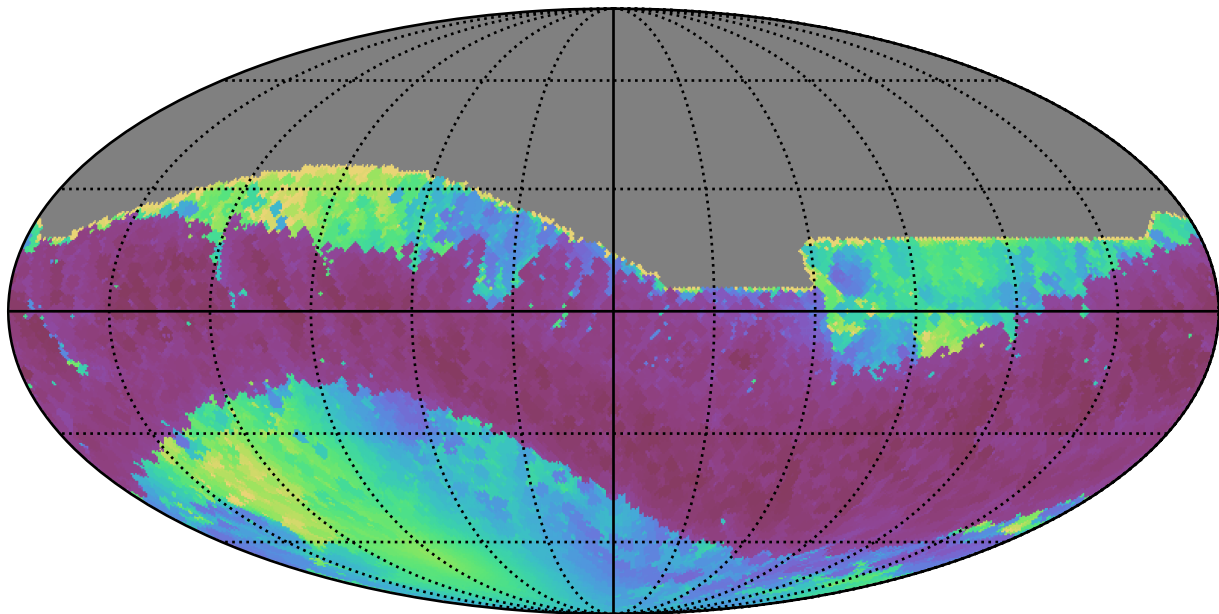
no_magell_roll_v3.4_10yrs All sky i band: Min solarElong
