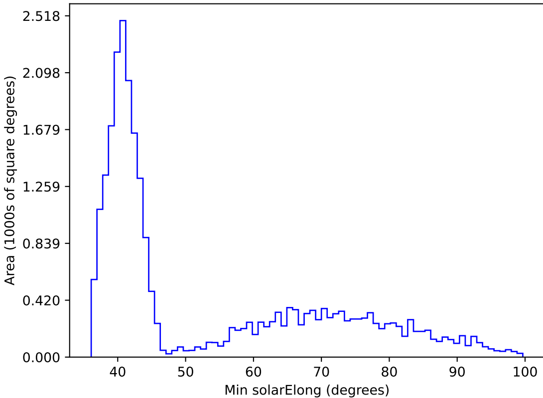
no_magell_roll_v3.4_10yrs All sky i band: Min solarElong
