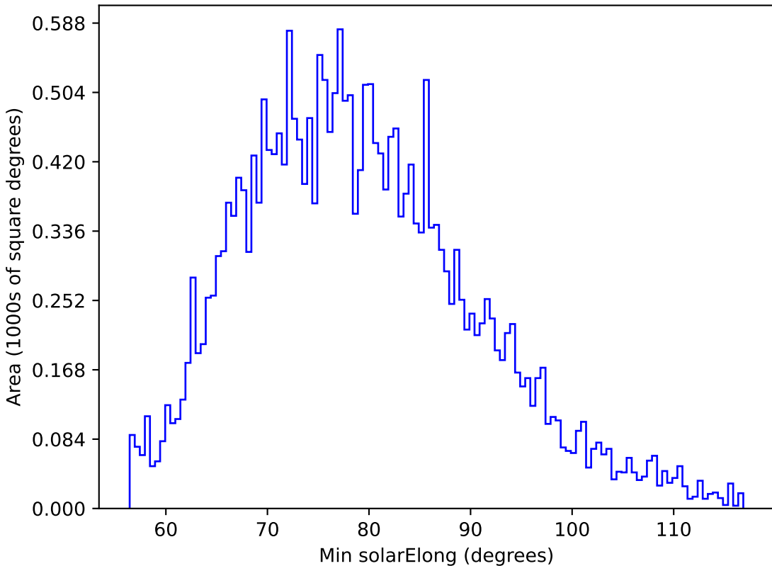
no_magell_roll_v3.4_10yrs All sky g band: Min solarElong
