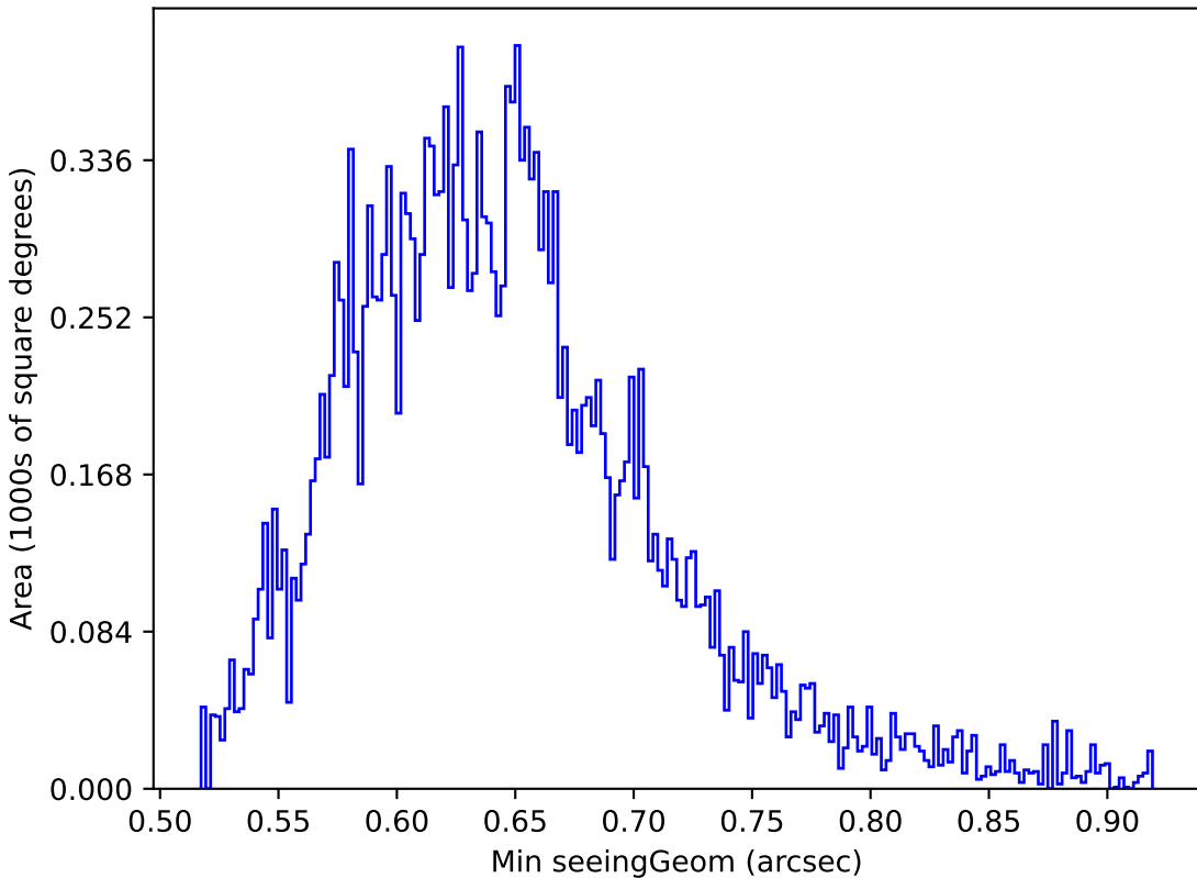
no_magell_roll_v3.4_10yrs Yr 1 y band: Min seeingGeom
