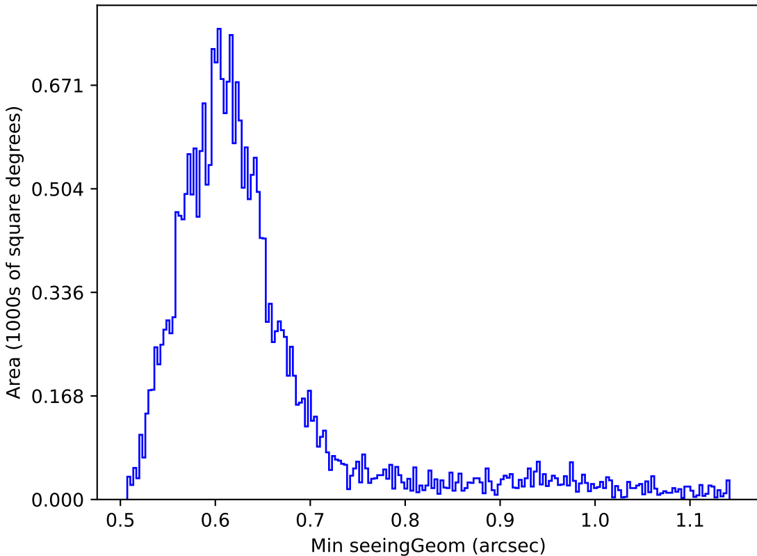
no_magell_roll_v3.4_10yrs Yr 1 r band: Min seeingGeom
