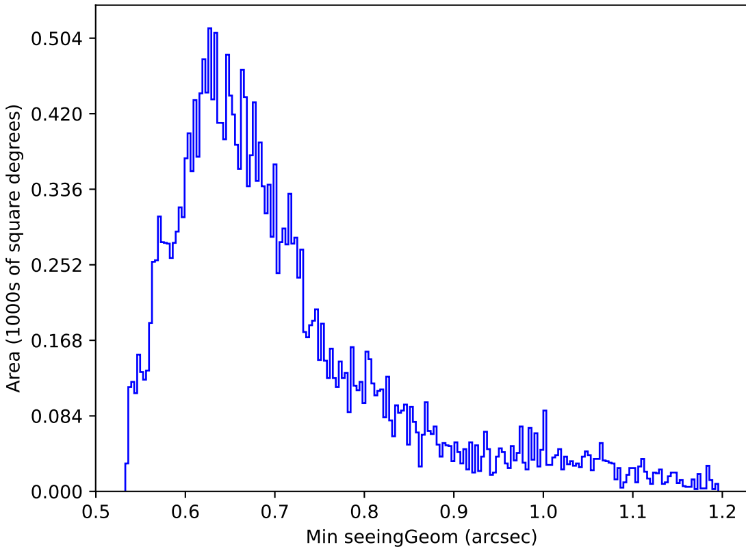
no_magell_roll_v3.4_10yrs Yr 1 g band: Min seeingGeom
