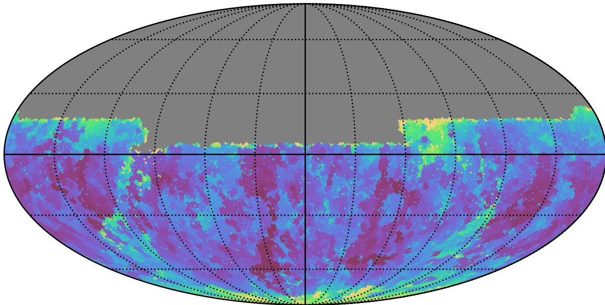
no_magell_roll_v3.4_10yrs Yr 1 y band: Min seeingEff
