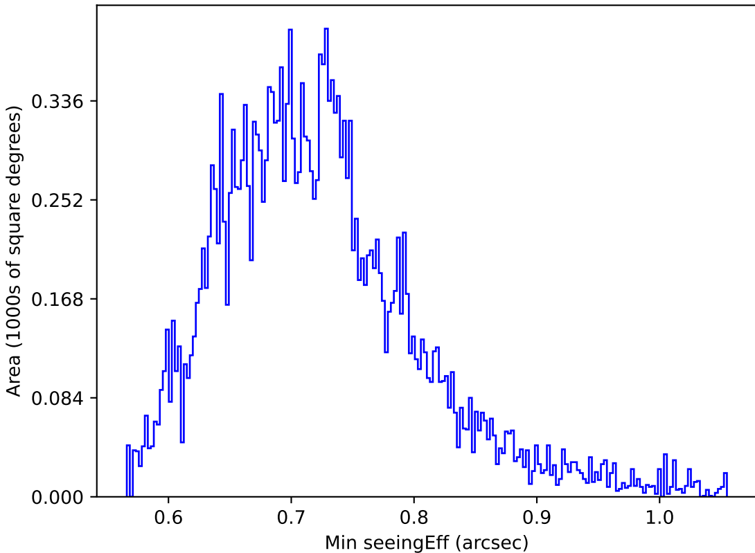
no_magell_roll_v3.4_10yrs Yr 1 y band: Min seeingEff
